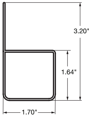
Rail Stiffener 018-4 $32.88/24'
