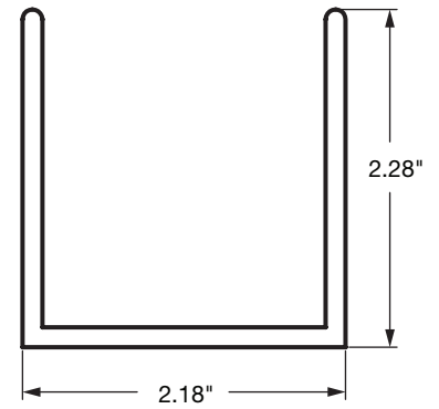
Rail Stiffener 018-6 $50.64/24'
